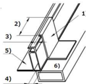
Abbildung 1. Anforderung an Klemmen (Clips)
