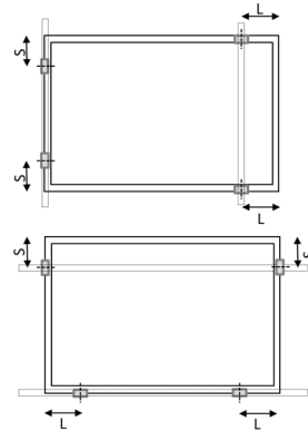
Bild B : Klemmenposition an kurzer und langer Rahmenseite
