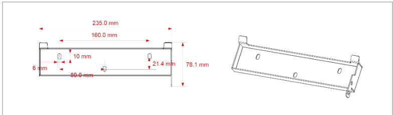
Abmessungen der Halterung für SOFAR 1.1K ... 3.3KTL-G3
