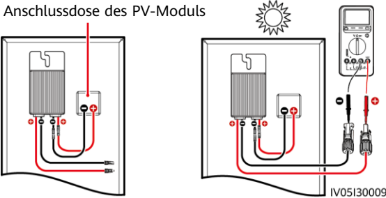
Anschlussdose des PV-Moduls
